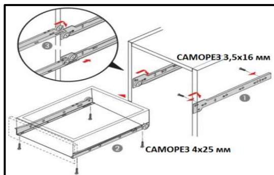
Рис. 1 Установка направляющих роликовых (установка на саморезы 3,5х16 и 4х25 мм)
